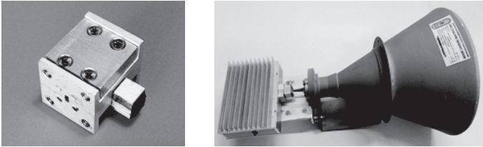
Рис. 6. Зовнішній вигляд підсилювача триміліметрового діапазону довжини хвилі (ліворуч) та приймального (передавального) тракту (праворуч)
