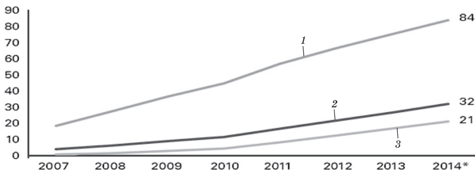
Рис. 1. Статистика пользователей подвижного ШПД — активных контрактов на 100 человек населения: 1 — развитые страны; 2 — в мире; 3 — развивающиеся страны
