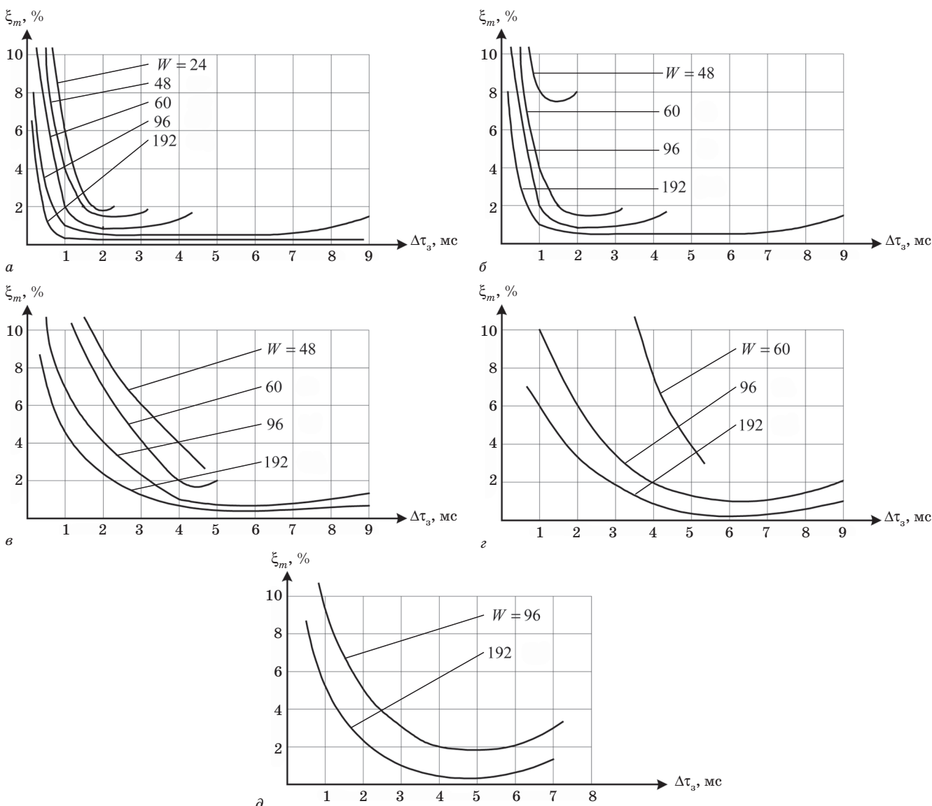
Рис. 1. Залежність \xi_m(\Delta\tau_3) при різних W для одного переприйомів ( a ); двох переприйомів ( б ); трьох переприйомів ( в ); чотирьох переприйомів ( г ) і п'яти переприйомів ( д )
